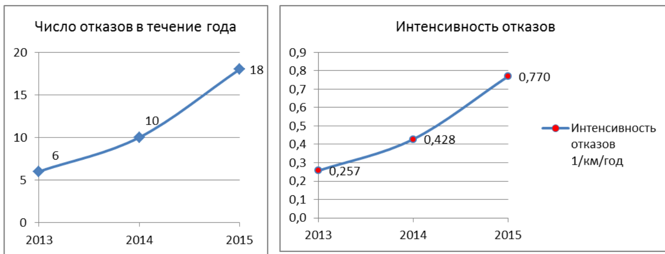
Рисунок 2.1.1.1. – Интенсивность отказов в зависимости от срока эксплуатации участка тепловой сети
