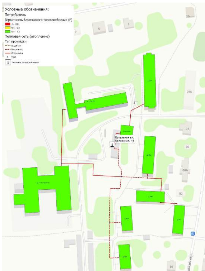
Рисунок 1.9.4.3 - Карта-схема зон надежности системы теплоснабжения котельной ул. Колхозная, 1В
