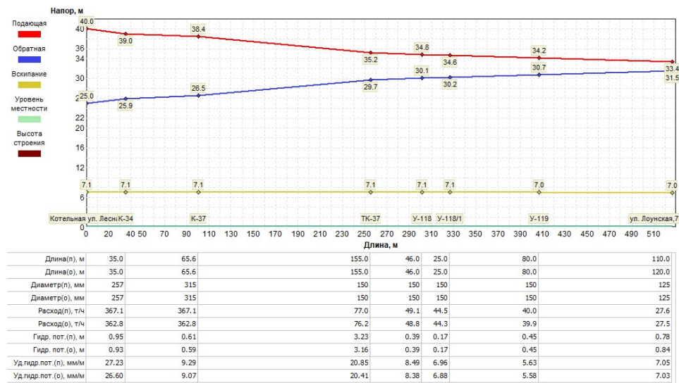
Рисунок 1.3.8.6 - Пьезометрический график участка сети Котельная ул. Лесная, 2 - ул. Лоунская, 7а, СОШ №1
