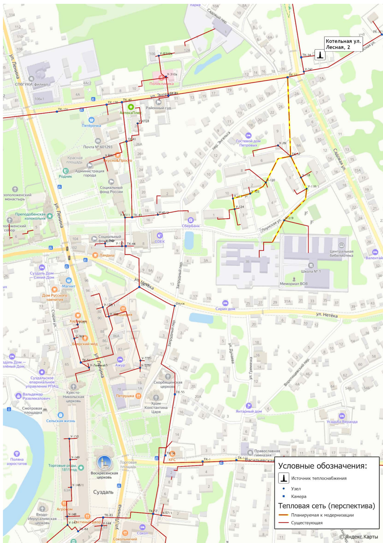
Рисунок 8.7.2 - Предложения по реконструкции (модернизации) тепловых сетей, подлежащих замене в связи с истечением эксплуатационного ресурса от котельной ул. Лесная, д.2
