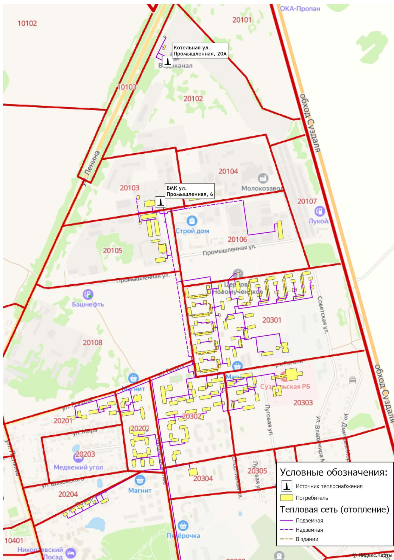
Рисунок 3.3.1 - Отображение объектов системы теплоснабжения БМК-16 МВт ул. Промышленная, 6 и котельной ул. Промышленная, 20А в границах кадастровых кварталов
