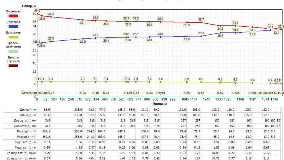
Рисунок 1.3.8.8 - Пьезометрический график участка сети Котельная ул. Лесная, 2 - ул. Ленина, 50, Индустр. колледж
