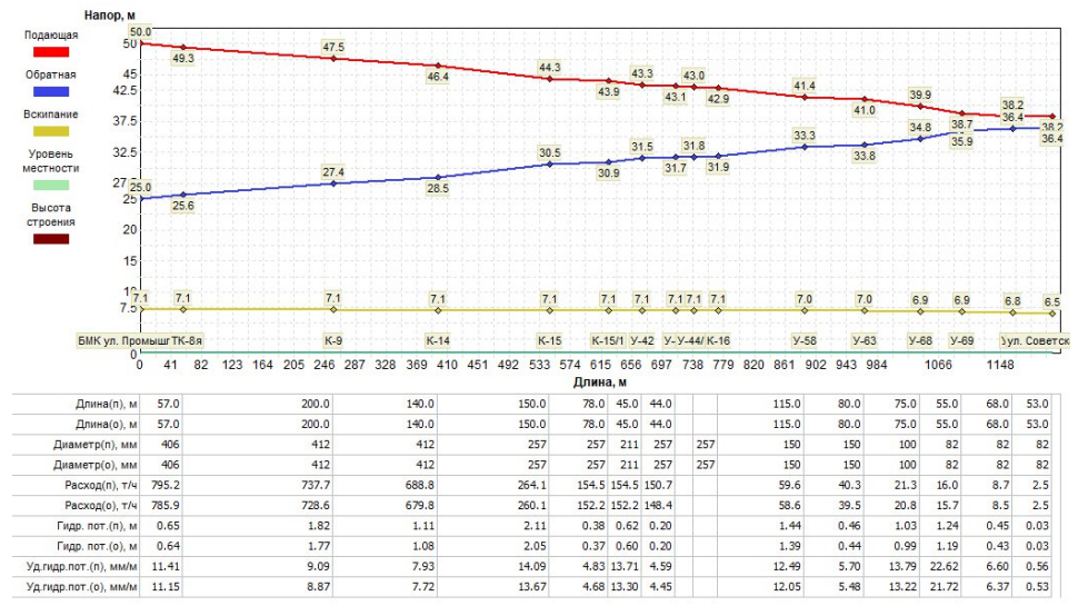
Рисунок 1.3.8.4 - Пьезометрический график участка сети БМК-16 МВт ул. Промышленная, 6 - ул. Советская, 58
