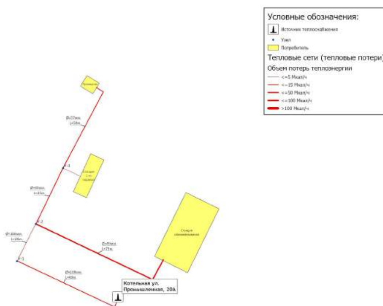
Рисунок 3.7.4 - Потери тепловой энергии при её передаче по участкам тепловых сетей от котельной ул. Промышленная, 20А
