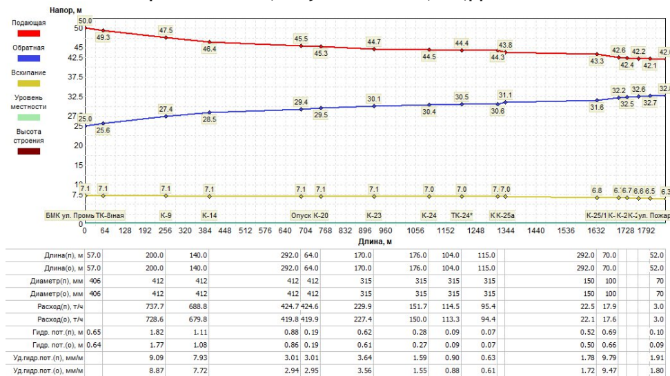
Рисунок 1.3.8.3 - Пьезометрический график участка сети БМК-16 МВт ул. Промышленная, 6 - ул. Пожарского, 4
