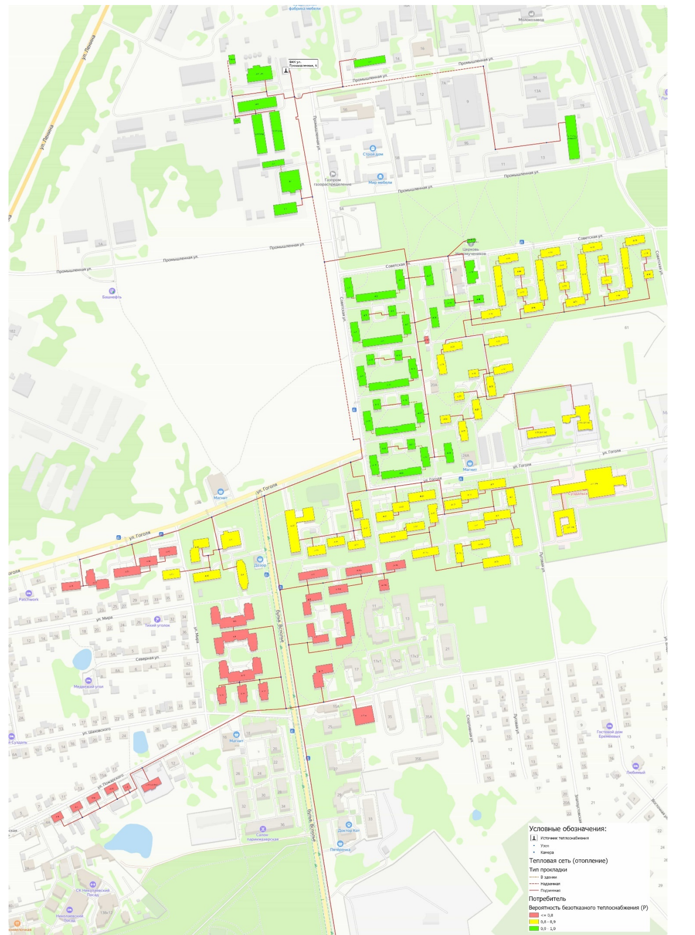
Рисунок 1.9.4.1 - Карта-схема зон надежности системы теплоснабжения БМК-16 МВт ул. Промышленная, 6
