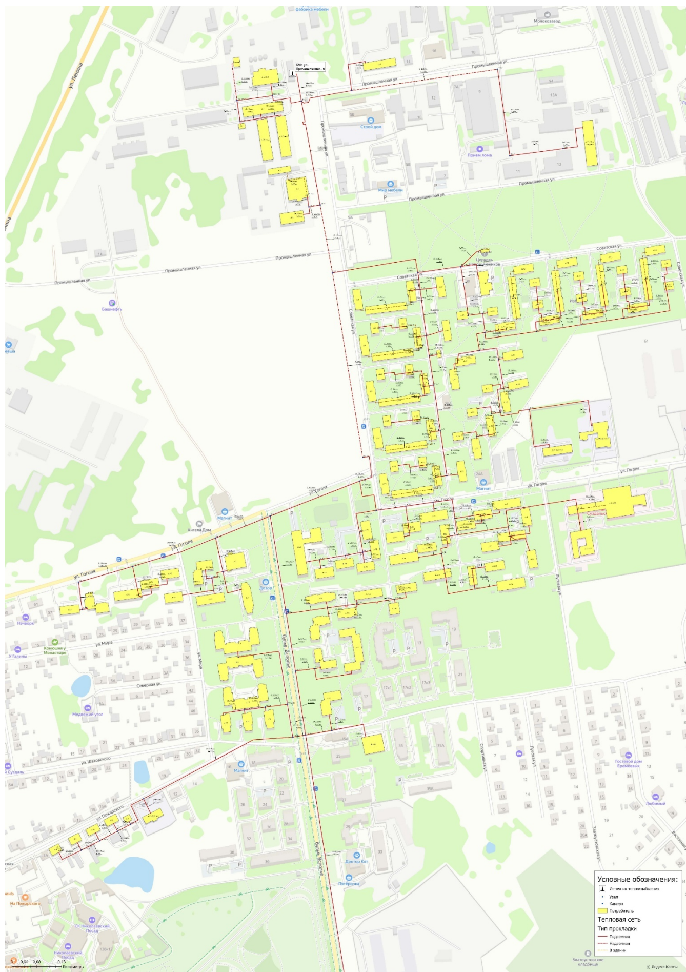
Рисунок 1.3.2.2 - Схема тепловых сетей БМК-16 МВт ул. Промышленная, 6
