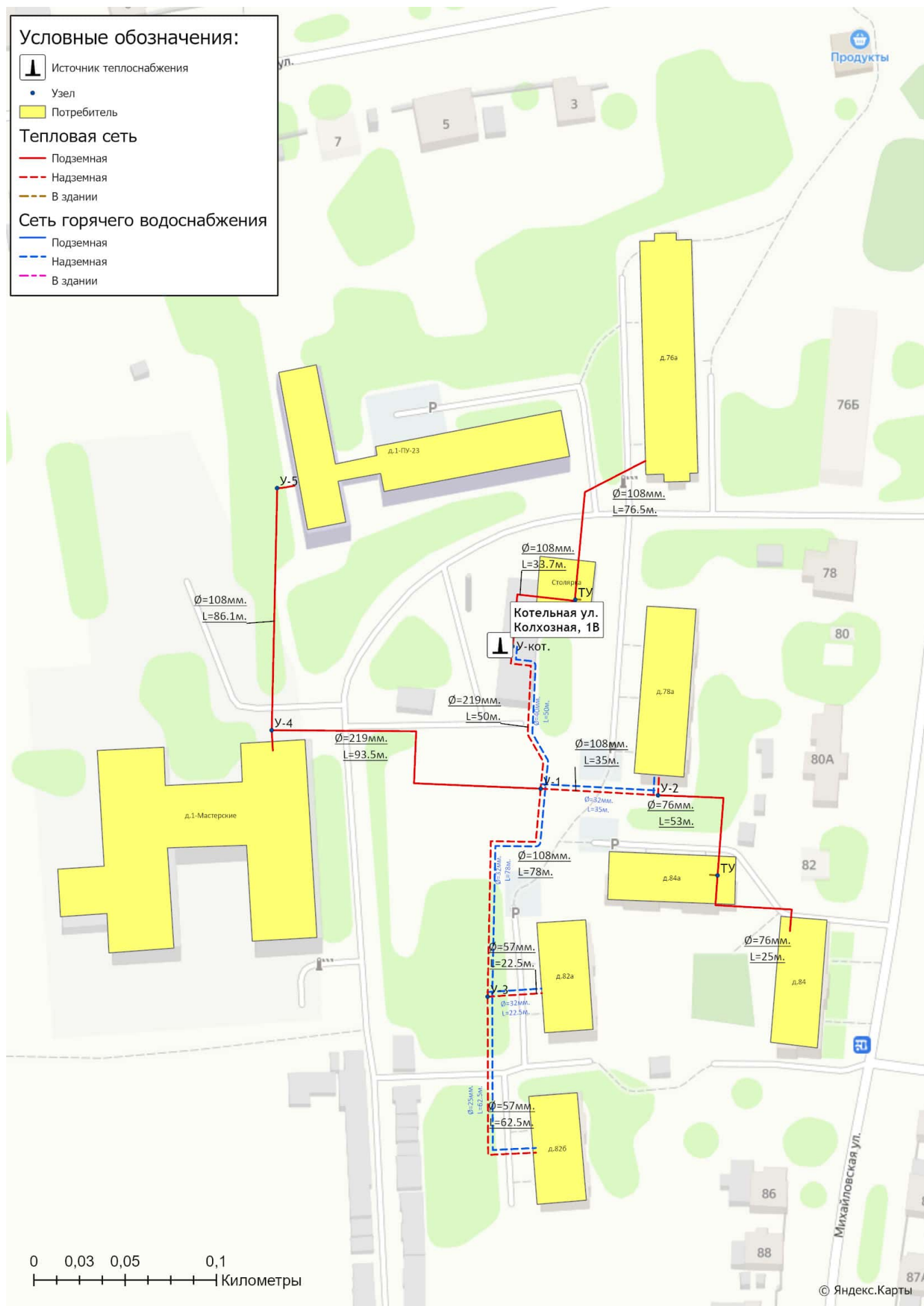
Рисунок 1.3.2.4 - Схема тепловых сетей котельной ул. Колхозная, 1В
