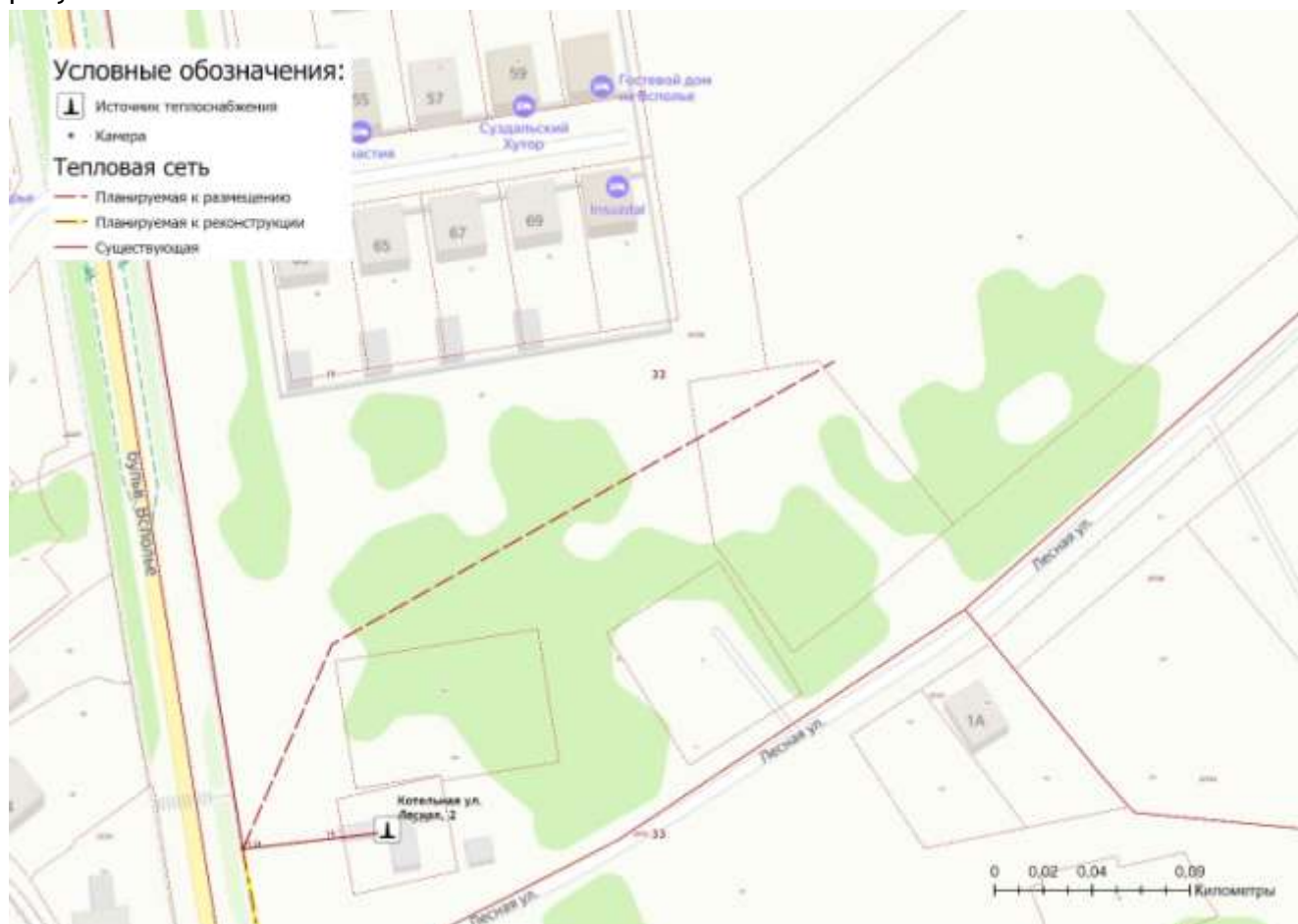
Рисунок 6.2.1 - Участок тепловых сетей для перспективного технологического присоединения потребителей по ул. Лесная, г. Суздаль
