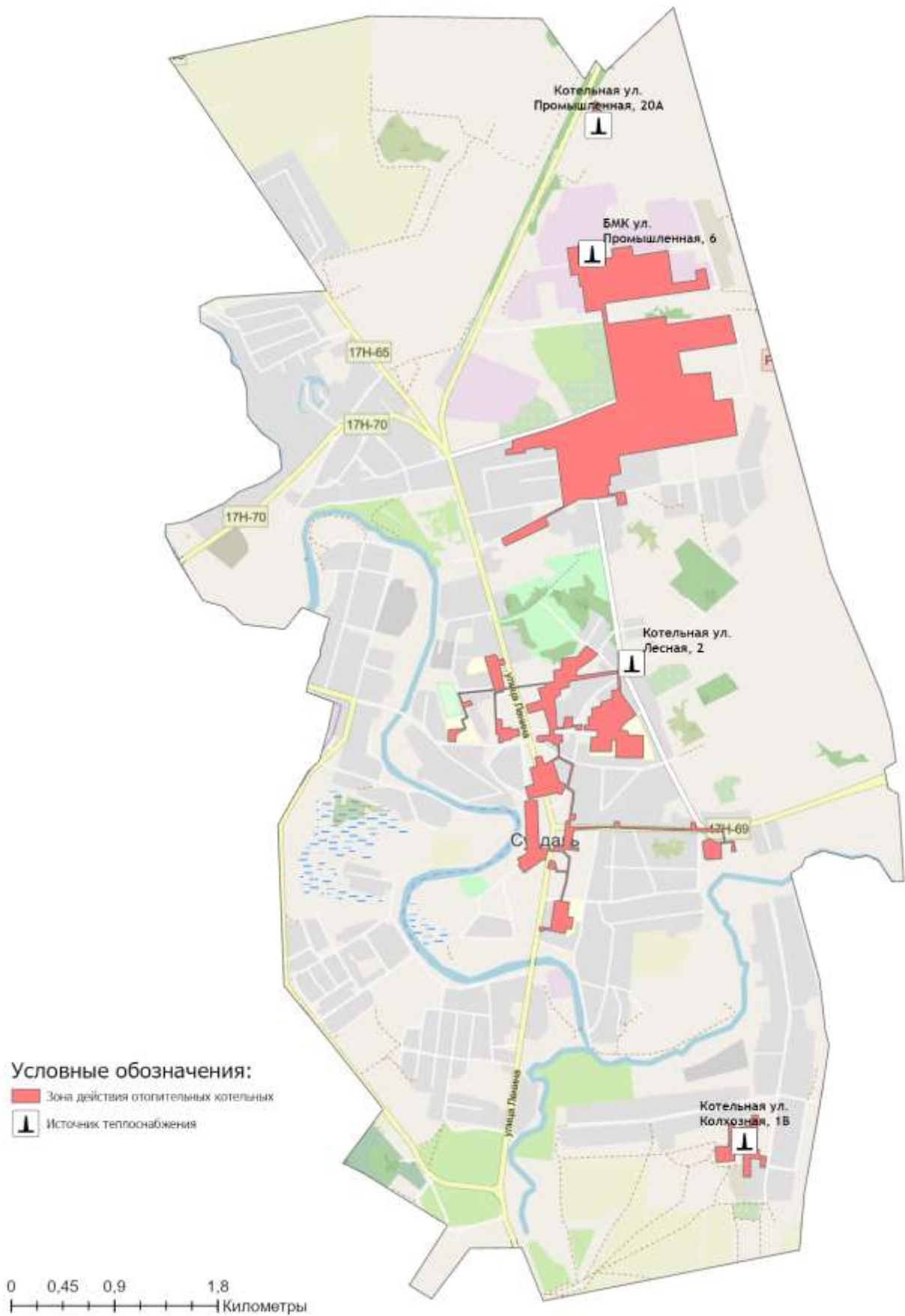
Рисунок 1.4.1 - Зоны действия централизованных систем теплоснабжения на территории муниципального образования город Суздаль
